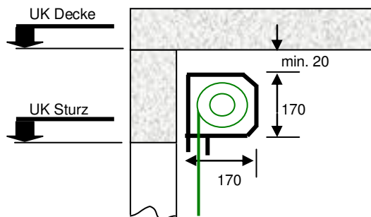
Schnitt B-B
