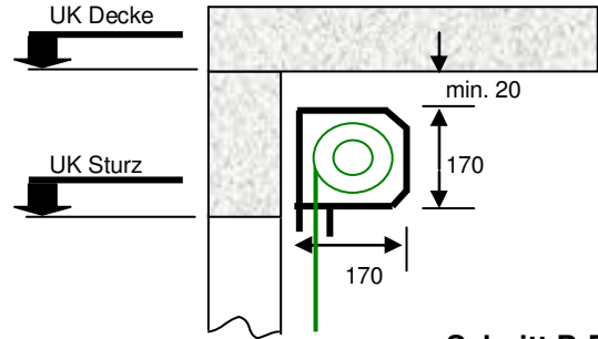
Schnitt B-B
